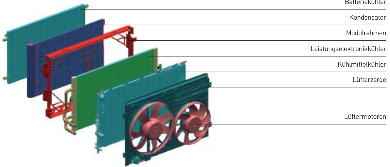
Kühlungskomponenten
